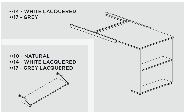
PIOLHP•• W 793 mm - H 90 mm - D 210 mm
